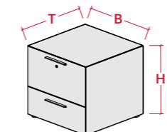
Einteilung 6-4 6 | 4 - Vollauszüge
