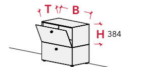
Aufsatz Modulschrank 1 OH - Klappe nach unten
