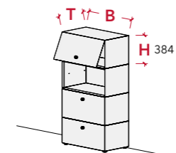
Aufsatz Modulschrank 1 OH - Klappe nach oben
